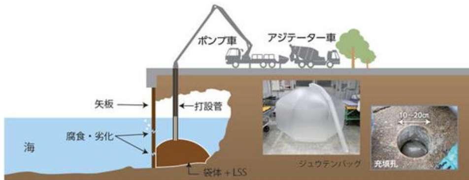
図-1 護岸でジュウテンバックを使用した施工イメージ
