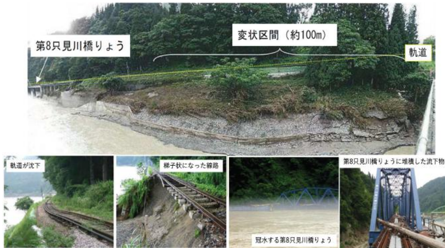
図-10 被災状況
