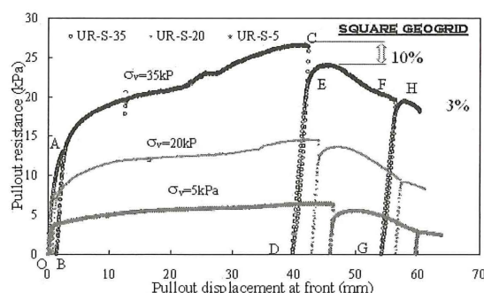
図-2 除荷・再載荷を含む引抜き試験結果
