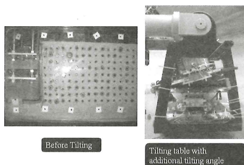
図-3 遠心傾斜台実験初期状態
