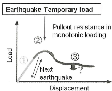
図-1 地震前～後の荷重条件の変化
