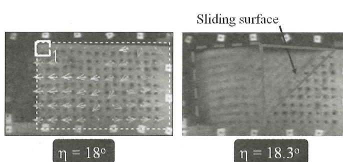
図-4 遠心傾斜台実験（再載荷による破壊）
