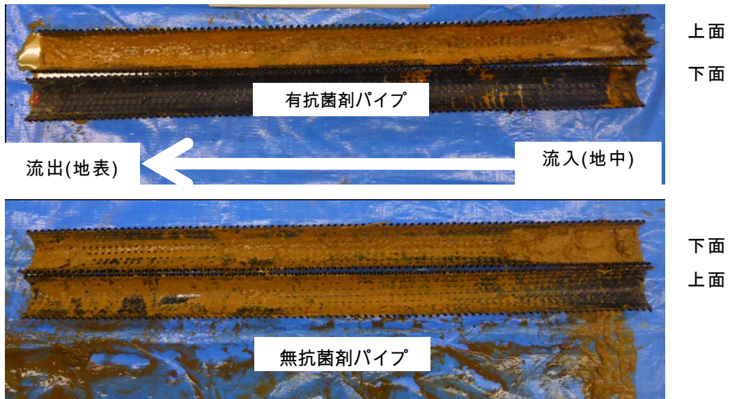
暗渠パイプ設置後の状況
