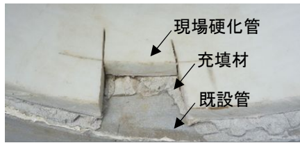
エアミルクの充填状況
