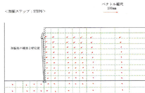
(b) 帯鋼補強土壁 Step6 828gal
