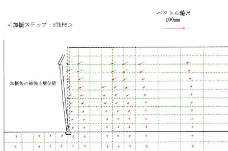
(a) 帯状ジオシンセティックス補強土壁 Step6 850gal
